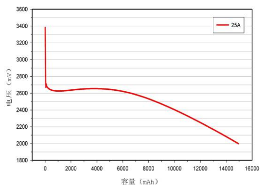
-10°C 1C低温放电曲线
