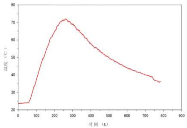
短路温度曲线
