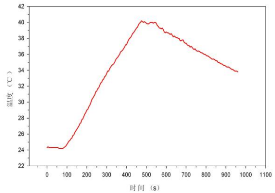
过充温度曲线
