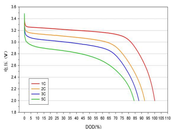
倍率放电曲线图
