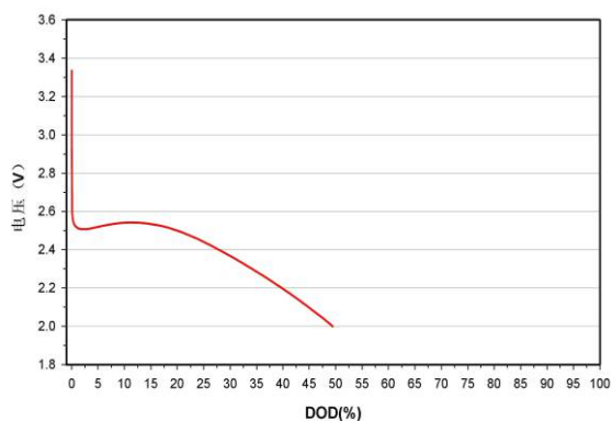
-20°C 1C低温放电曲线
